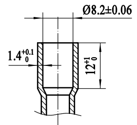
排气管放大图 Discharge Tube (Scaled)
